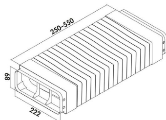
Easy-Fix Rektangulær fleksibel slange
