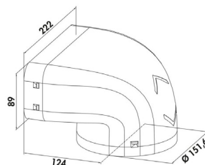
Easy-Fix Rektangulær bend til sirkulær Ø150
