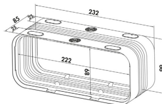
Easy-Fix Fast rektangulært skjøtestykke
