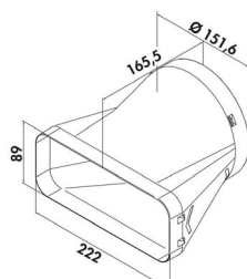
Easy-Fix Overgang rekt. til sirk. Ø150
